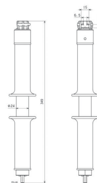
Maßbild
