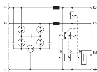
Prinzipschaltbild
