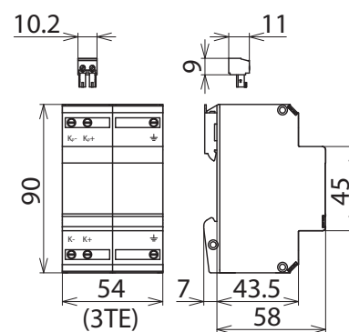
Maßbild
