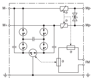
Prinzipschaltbild
