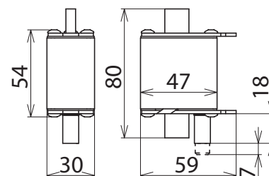
Maßbild
