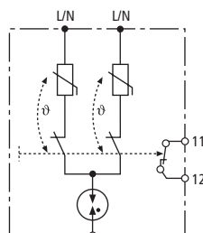
Prinzipschaltbild
