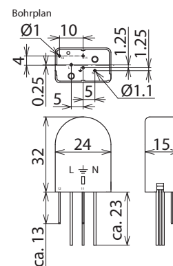
Maßbild
