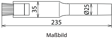
Maßbild
