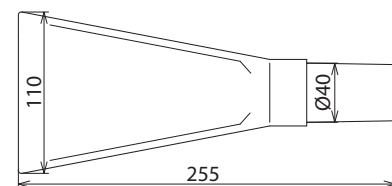
Maßbild
