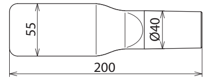
Maßbild
