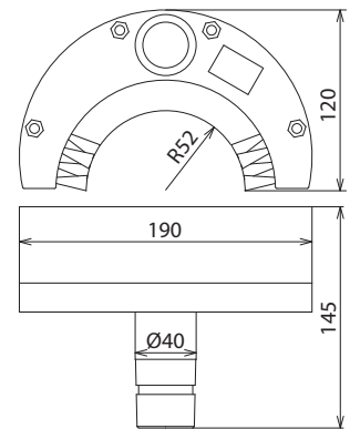
Maßbild
