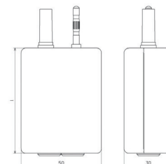
Maßbild
