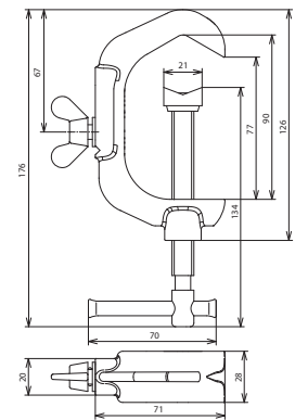
Maßbild
