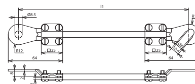
Maßbild
