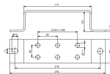
Maßbild
