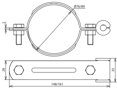
Maßbild
