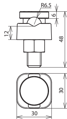
Maßbild
