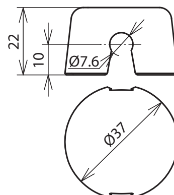
Maßbild
