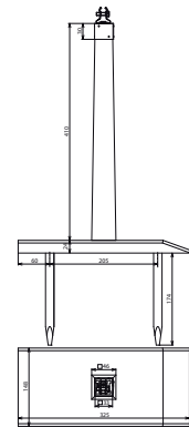
Maßbild
