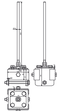
Maßbild
