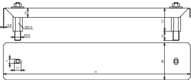
Maßbild
