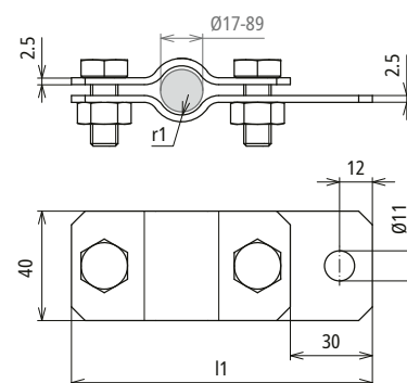
Maßbild
