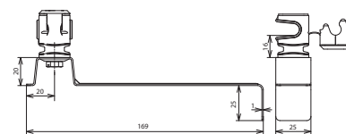
Maßbild
