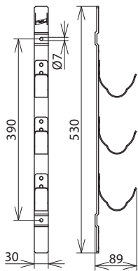
Maßbild
