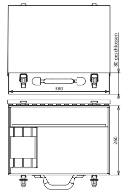
Maßbild
