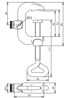
Maßbild
