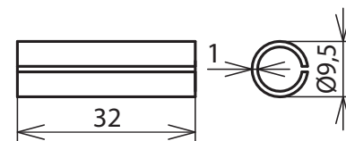
Maßbild
