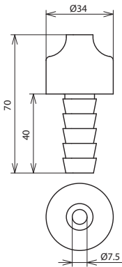
Maßbild
