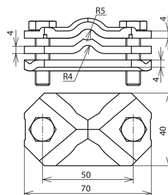
Maßbild
