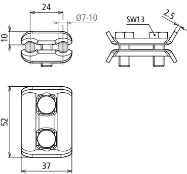
Maßbild
