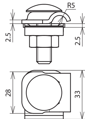
Maßbild
