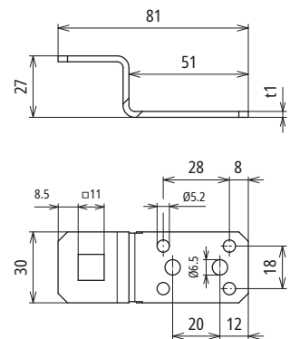
Maßbild
