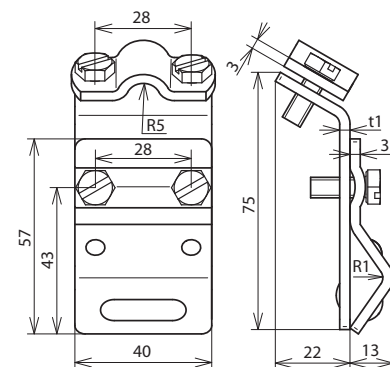
Maßbild
