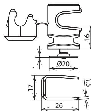
Maßbild
