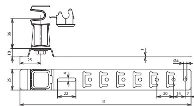
Maßbild
