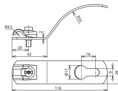
Maßbild
