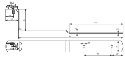
Maßbild
