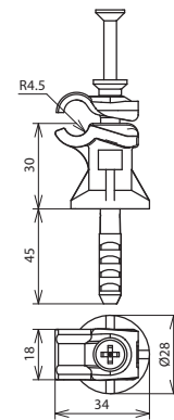
Maßbild
