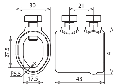
Maßbild
