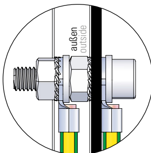
Variante 1: Anschluss außen variant 1: connection outside
