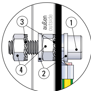
Auslieferungszustand delivery status
