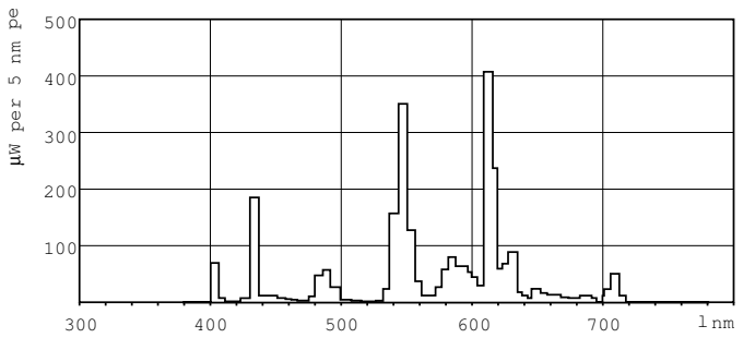
Lichtfarbe /830
