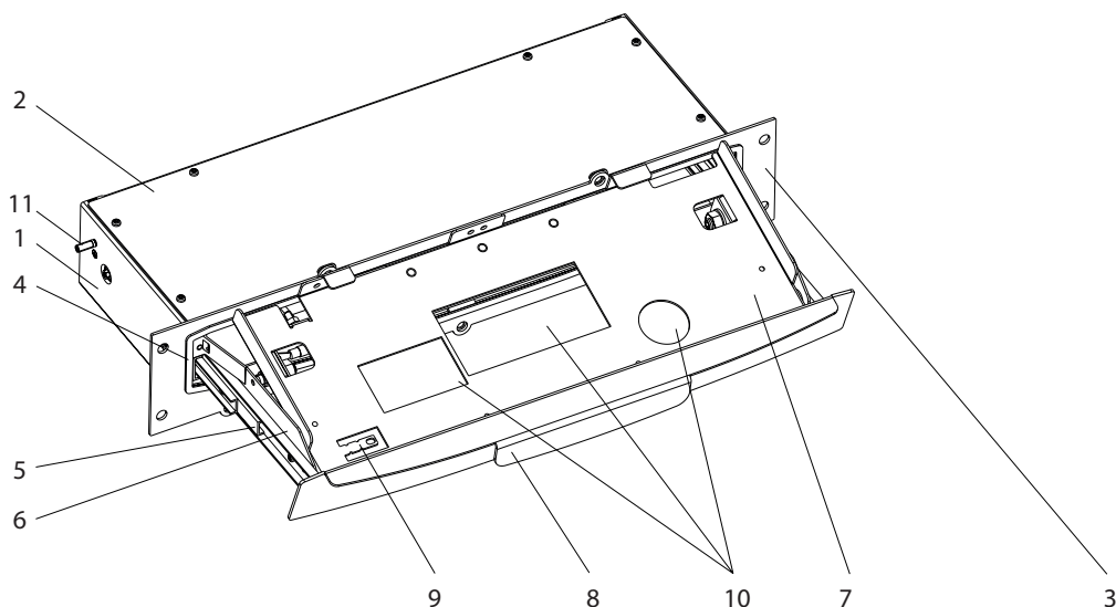
Abbildung C: Schublade geöffnet und 20° geschwenkt
