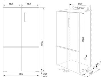
MD53NOCH (ohne Wasseranschluss)
