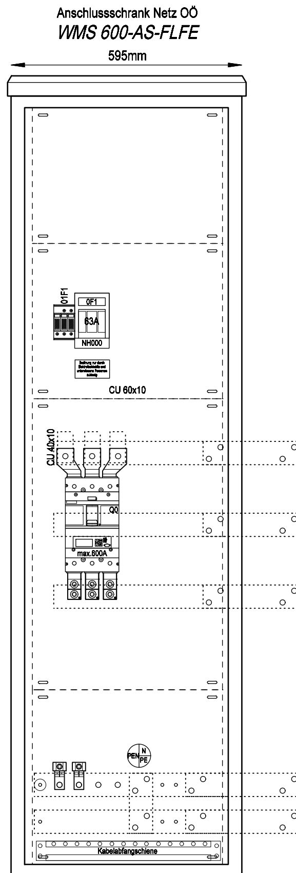
FL-B-U/1/AL Frontansicht ohne Tür
