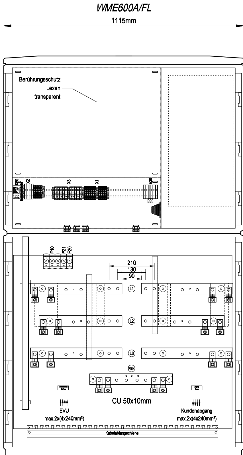
Frontansicht ohne Tür
