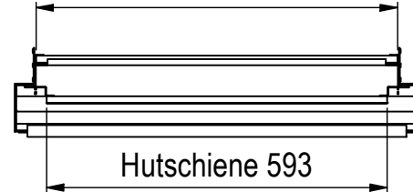
Hutschiene Vorzählerfach 629
