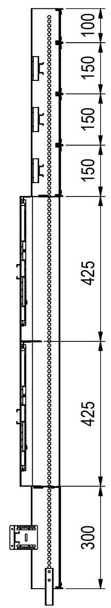
A-A ( 1 : 11 )
