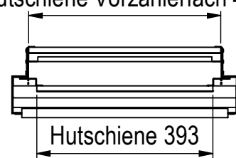
Hutschiene Vorzählerfach 429
