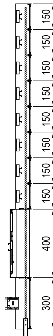
A-A ( 1 : 13 )
