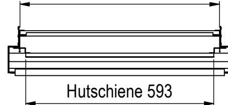
Hutschiene Vorzählerfach 629
