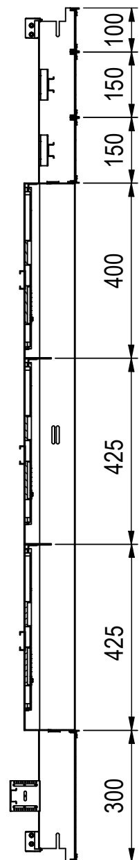
A-A ( 1 : 12 )
