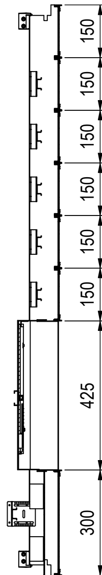
A-A ( 1 : 11 )
